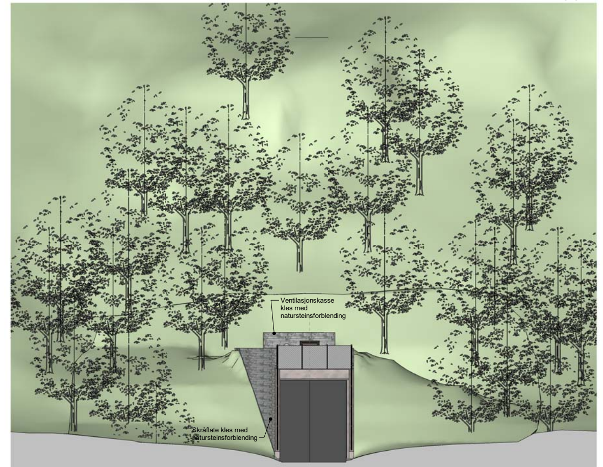
Oppriss/fasade vest 1 : 100
